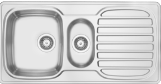
H 971 K Art. nr. 80542085 RSK nr. 8018242 60 Stor låda 340x400x160 Liten låda 160x295x120 Ytermått 971x496
