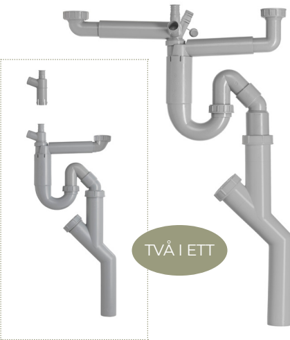
Vattenlås Universal ROT Art. nr 8992080 RSK nr 8124256 Vattenlås med teleskopsarmar, anpassningsbart både för dubbel och enkelho montage. Dimension G40x50mm.
