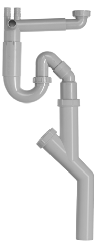
Vattenlås för enkellåda ROT Art. nr 8993080 RSK nr 8084755 Vattenlås för enkellåda med teleskopsarm samt fyra maskinuttag. Dimension G40x50mm.
