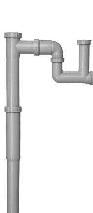
Vattenlås för enkellåda med teleskopsrör Art. nr 8800080 RSK nr 8084725 Komplett vattenlås för enkellåda med rakt teleskopsrör. Dimension G40x50mm.
